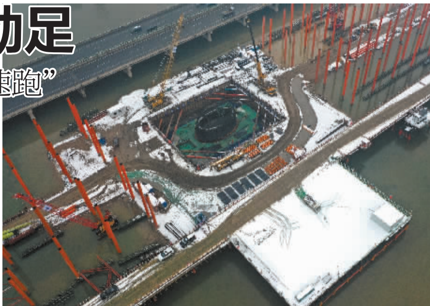
■滹沱河特大桥项目现场,施工人员进行主墩承台施工。
